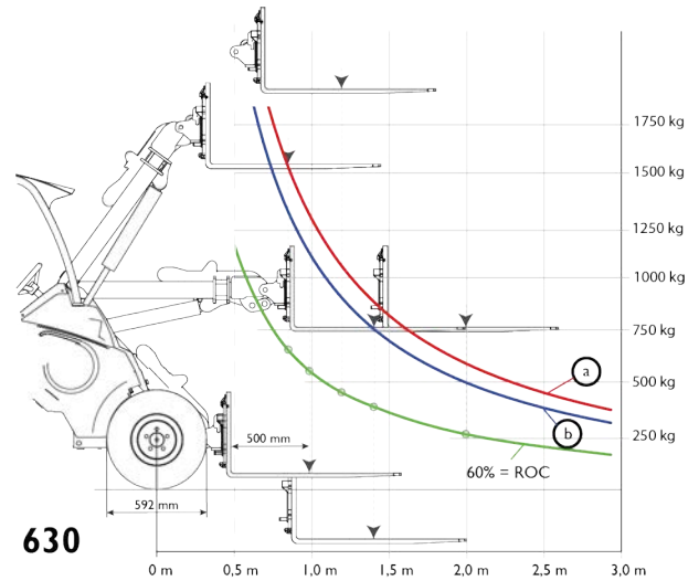
Belastningsdiagram 630/635/640
